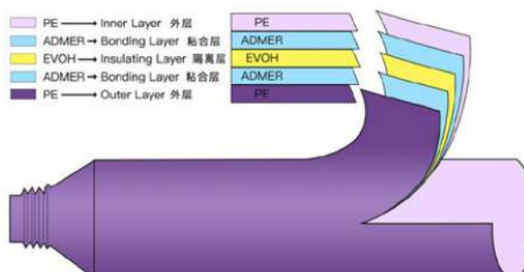
b. Five-layer PE tube 5层PE管
